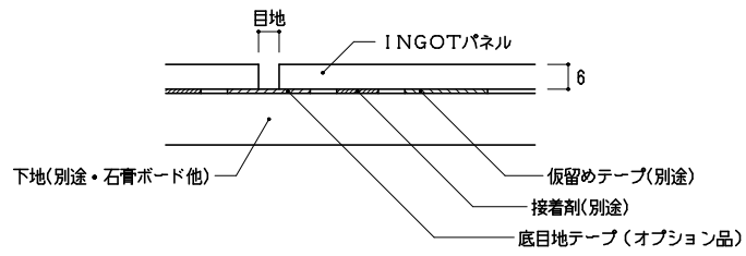
平目地部分
