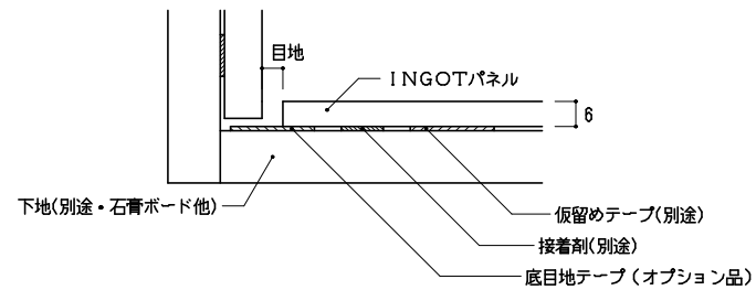
入隅部分
