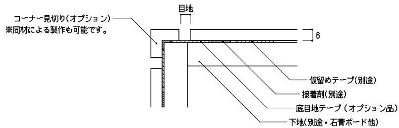
出隅部分
