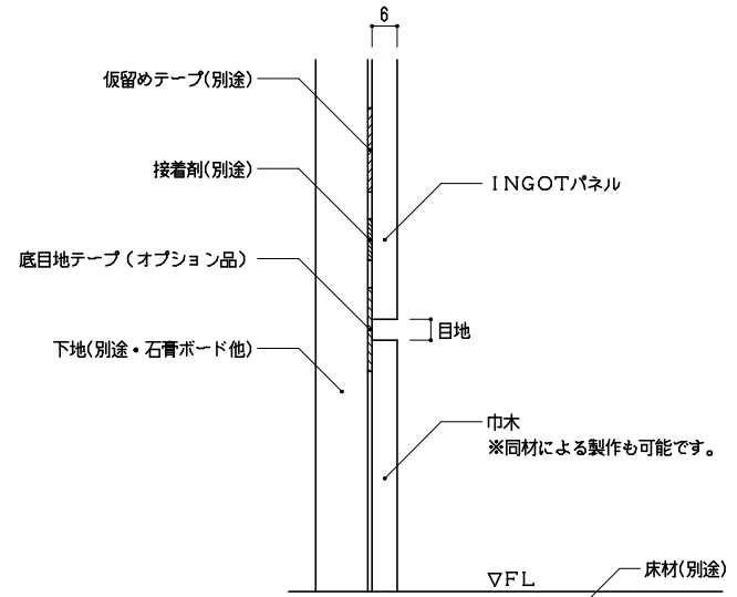
巾木部分
